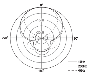
POLÆRT MØNSTER
