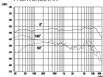
FREKVENSSVAR
